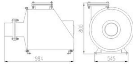
Blower B-2000LN
